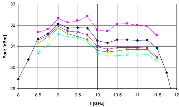
Output power ( V_d=8V , V_{g1}=-5V , P_s=17dBm )
